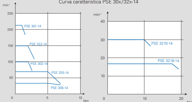
Curva caratteristica PSE 30x/32x-14
