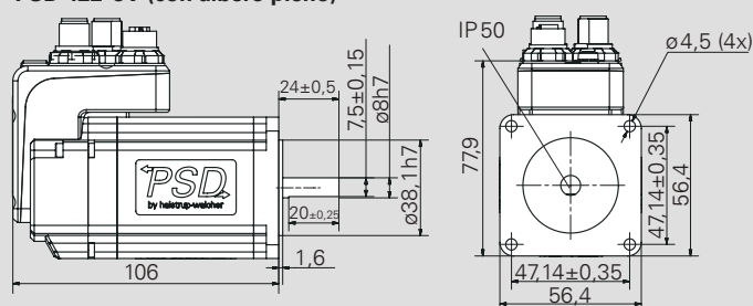
PSD 432-8/14H (con albero cavo, 2 Nm)
