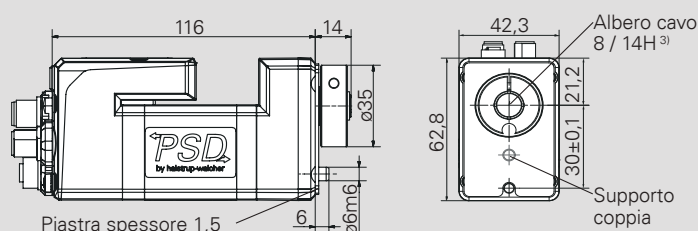
PSD 413-8/14H (con albero cavo, 3 Nm)
