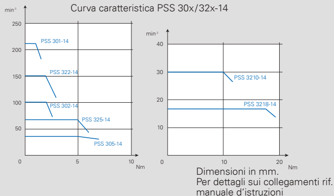
Curva caratteristica PSS 30x/32x-14
