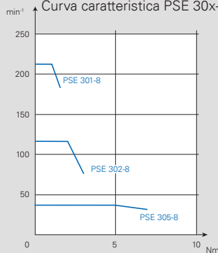
Curva caratteristica PSE 30x-8
